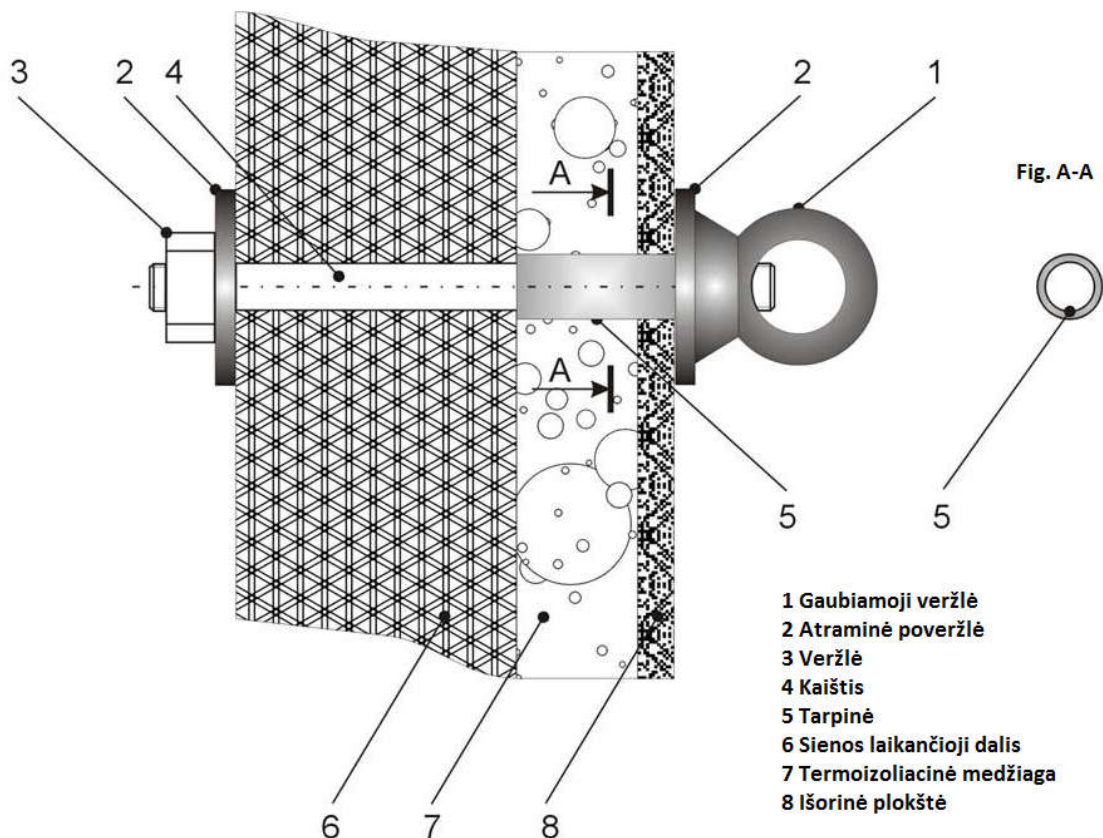
7 pav. Montavimo schema
