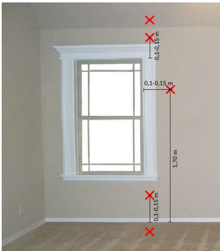
4 pav. Rekomenduojami STT montavimo taškai pastato viduje
