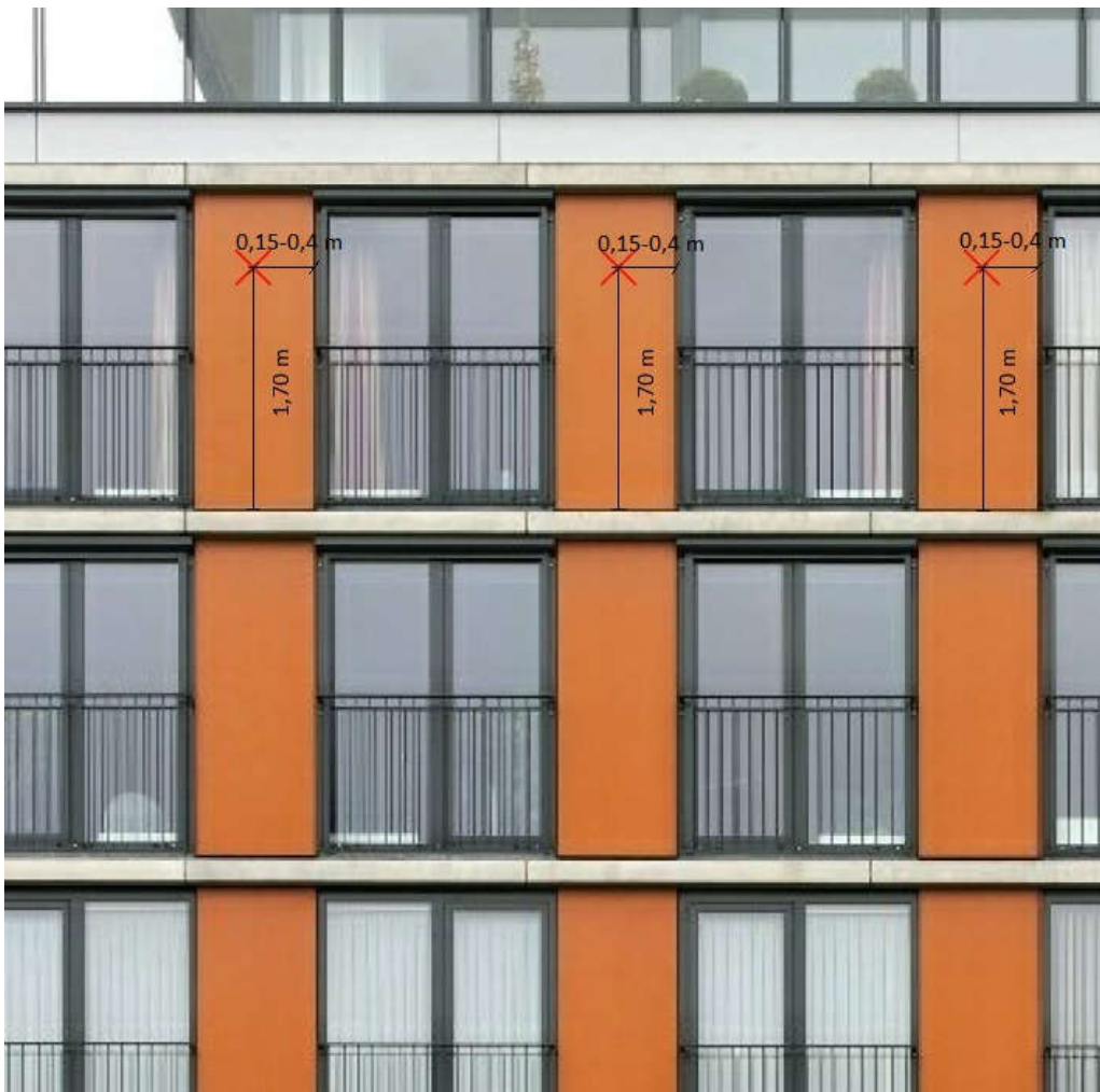
2 pav. Stacionaraus taško montavimas išorėje
